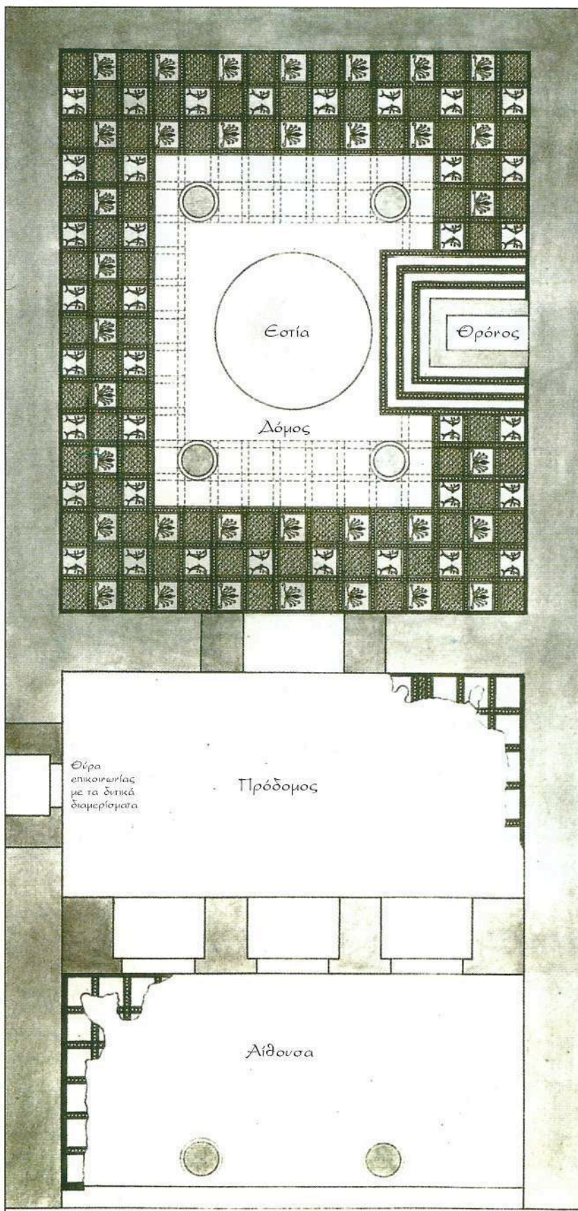
Σχεδιαστική αναπαράσταση του δαπέδου του μεγάλου μεγάρου του ανακτορίου της Τίρυνθας (της αίθουσας, του προδόμου και του δόμου), κατά τους G. Rodenwaldt και Π. Σούρτσο.
