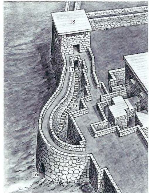
Αναπαράσταση του δυτικού προμαχώνα, με τον ΒΑ πύργο [αρ. 18], το μεγάλο κλιμακοστάσιο [αρ. 15] και την πυλίδα [αρ. 16] (Konstantinos Kontorlis, Mycenaean Civilization. Mycenae - Tiryns - Asine - Midea - Pylos, Athens 1985, p. 64 ).
