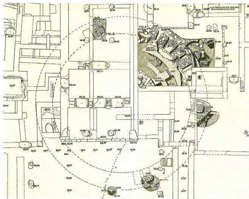
Κάτοψη του Κυκλικού Οικοδομήματος της Τίρυνθας, χρονολογούμενο κατά την Πρωτοελλαδική ΙΙ (2400-2300 π.Χ.), κάτω από το μεταγενέστερο μυκηναϊκό μέγαρο στην άνω ακρόπολη.
