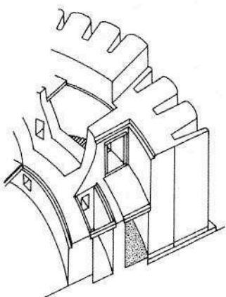
Προοπτική αναπαράσταση του σωζόμενου τμήματος του Κυκλικού Οικοδομήματος της Τίρυνθας (κατά P. Haider).
